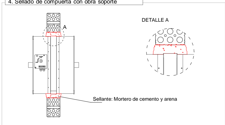
4. Sellado de compuerta con obra soporte
