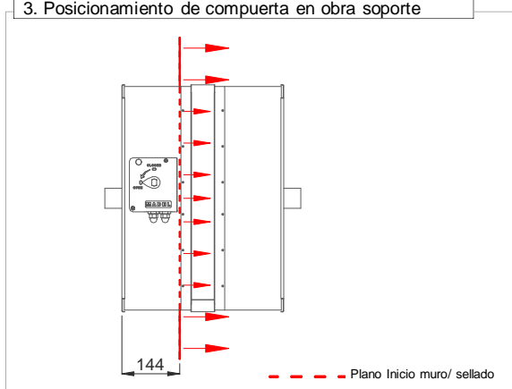
3. Posicionamiento de compuerta en obra soporte
