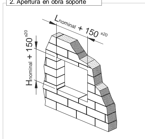
2. Apertura en obra soporte
