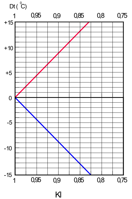
FACTEUR DE CORRECTION DE LA PORTÉE (L0,2) DT (-).
