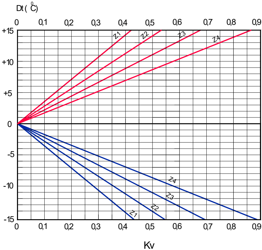
FACTEUR DE CORRECTION POUR LA DIFFUSION VERTICALE (bv) POUR DT (-).
