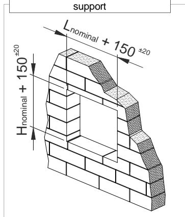
1. Ouverture dans chantier support
