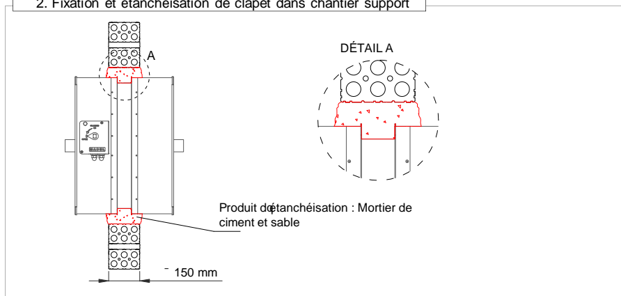
2. Fixation et étanchéisation de clapet dans chantier support
