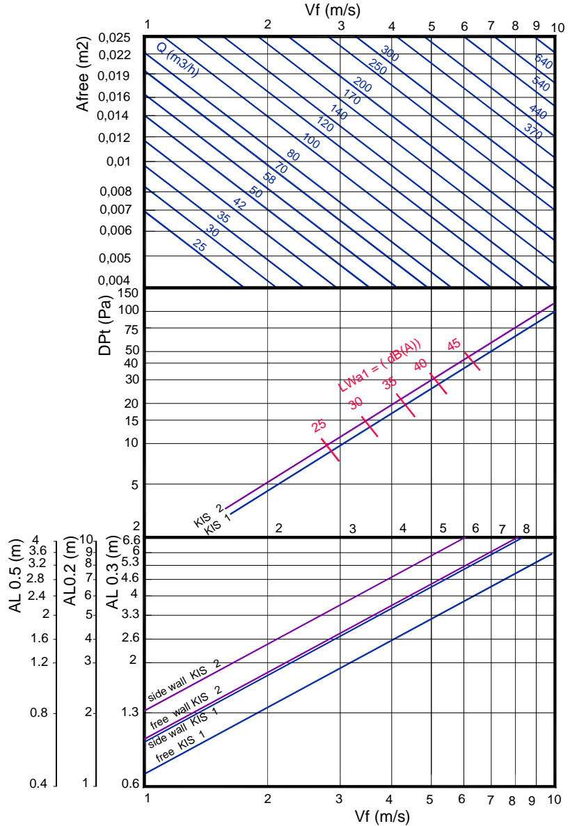
FACTOR DE CORRECCION DEL ALCANCE KL
