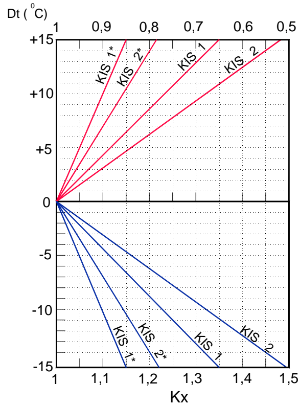
FACTOR DE CORRECCION DEL ALCANCE VERTICAL ( AL_{0,2} ) DT
