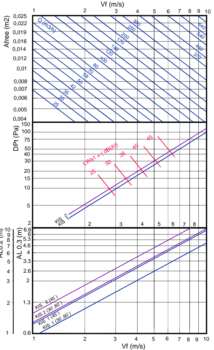
VALORES DE CORRECCION PARA Dpt Y Lwa1.
